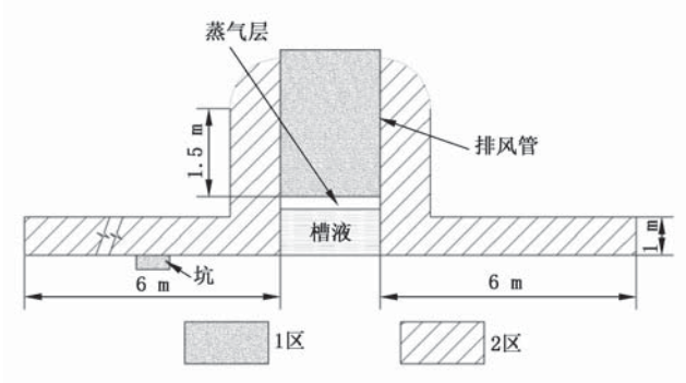
b) 有蒸气控制和通风
