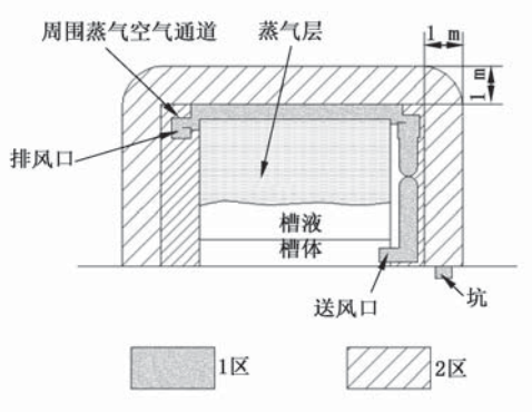
b) 有蒸气控制和通风
