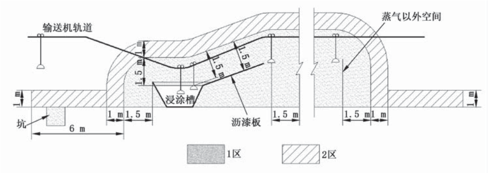
a) 无蒸气控制或通风
