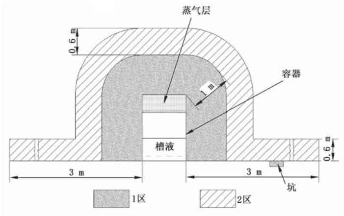
图 A.3 通风区域开放式容器周围浸涂爆炸性气体环境危险区域划分图
